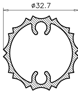
1.366 PESO TCO: 0.548 PERIMETRO: 0.24
