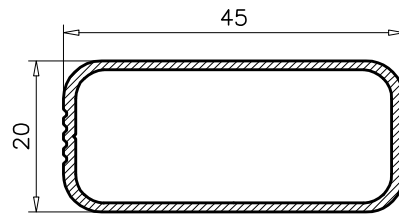
7.816 PESO TEORICO: 0.413 PERIMETRO: 0.24
