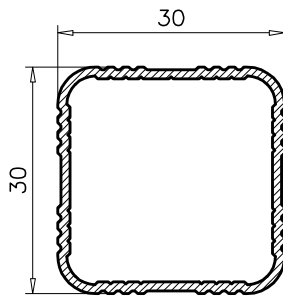
7.815 PESO TEORICO: 0.378 PERIMETRO: 0.23
