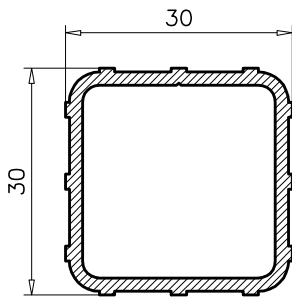
1.901 PESO TEORICO: 0.521 PERIMETRO: 0.22
