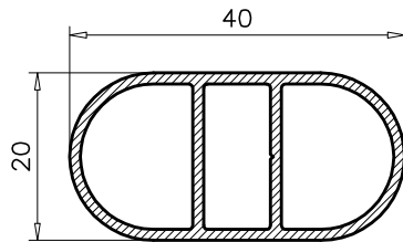
6.334 PESO TEORICO: 0.470 PERIMETRO: 0.26
