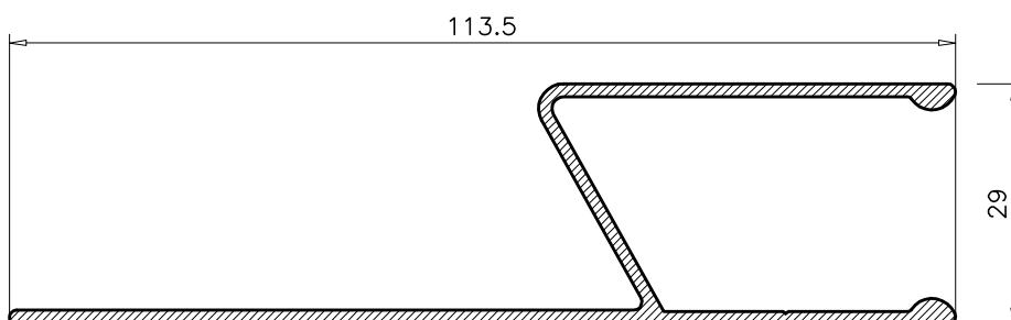
7.682 PESO TEORICO: 0.974 PERIMETRO: 0.39
