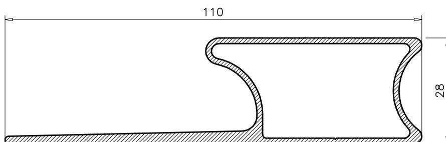
7.680 PESO TEORICO: 1.268 PERIMETRO: 0.44
