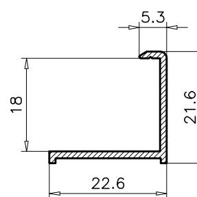
6.123 PESO TEORICO: 0.165 PERIMETRO: 0.10
