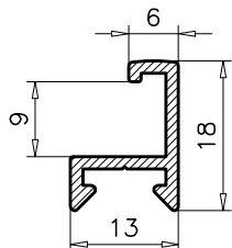
2.727 PESO TEORICO: 0.170 PERIMETRO: 0.10
