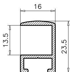
5.793 PESO TEORICO: 0.257 PERIMETRO: 0.13
