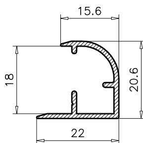
5.997 PESO TEORICO: 0.213 PERIMETRO: 0.12
