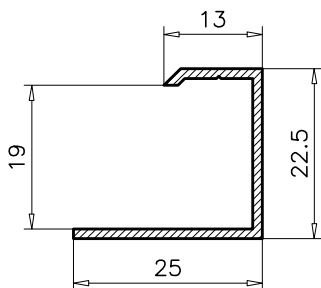
4.862 PESO TEORICO: 0.203 PERIMETRO: 0.12
