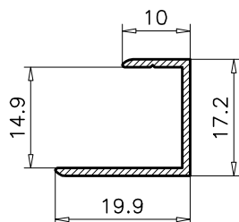
9.864 PESO TEORICO: 0.156 PERIMETRO: 0.10
