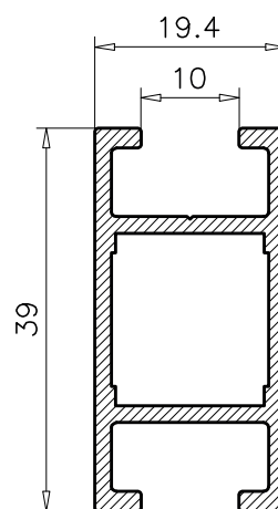
9.436 PESO TEORICO: 0.632 PERIMETRO: 0.24
