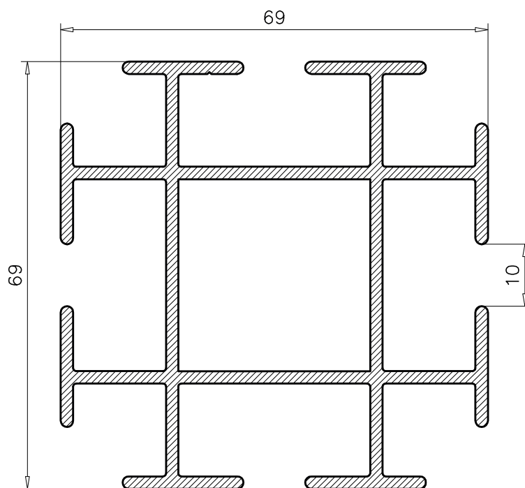
9.437 PESO TEORICO: 2.354 PERIMETRO: 0.80
