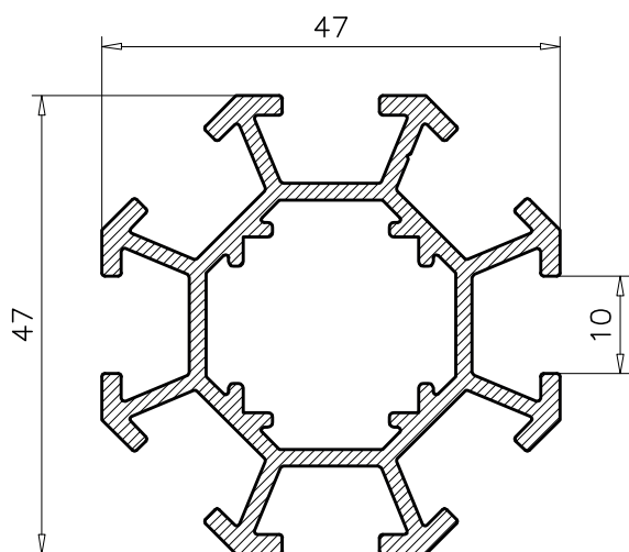
9.435 PESO TEORICO: 1.243 PERIMETRO: 0.46
