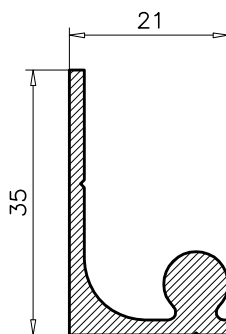
5.162 PESO TEORICO: 0.122 PERIMETRO: 0.10
