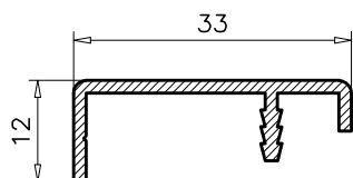
5.164 PESO TEORICO: 0.232 PERIMETRO: 0.12
