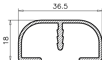
5.468 PESO TEORICO: 0.346 PERIMETRO: 0.19
