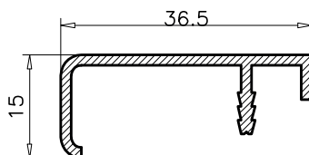
4.439 PESO TEORICO: 0.270 PERIMETRO: 0.14
