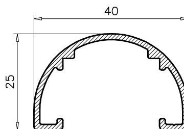
5.230 PESO TEORICO: 0.383 PERIMETRO: 0.18
