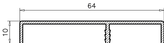
6.873 PESO TEORICO: 0.327 PERIMETRO: 0.18
