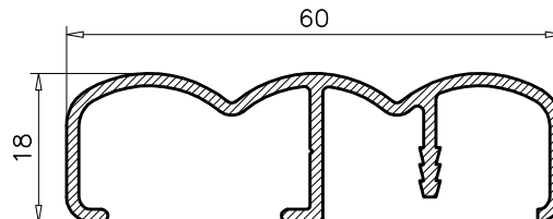
5.934 PESO TEORICO: 0.518 PERIMETRO: 0.25
