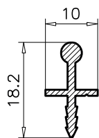
4.143 PESO TEORICO: 0.122 PERIMETRO: 0.10
