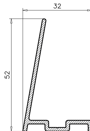
6.178 PESO TEORICO: 0.421 PERIMETRO: 0.19
