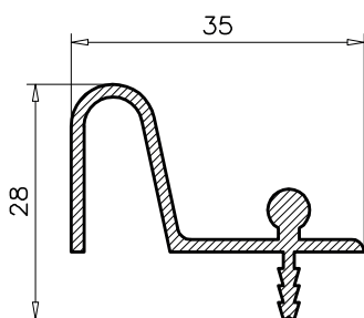
4.025 PESO TEORICO: 0.362 PERIMETRO: 0.17
