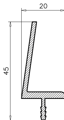
4.667 PESO TEORICO: 0.381 PERIMETRO: 0.13
