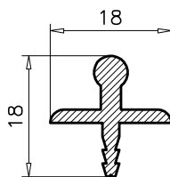
4.024 PESO TEORICO: 0.216 PERIMETRO: 0.10
